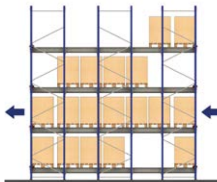
Systém FIFO
